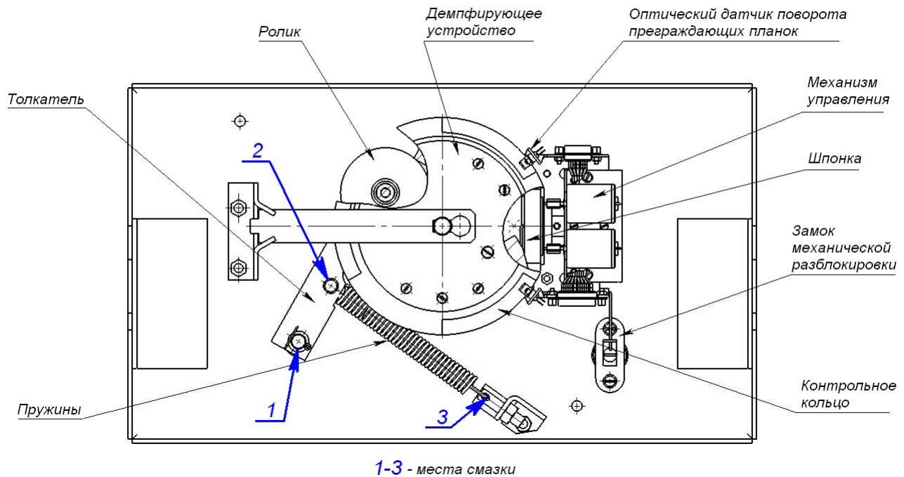
Рисунок 13. Расположение внутренних деталей и узлов стойки турникета
