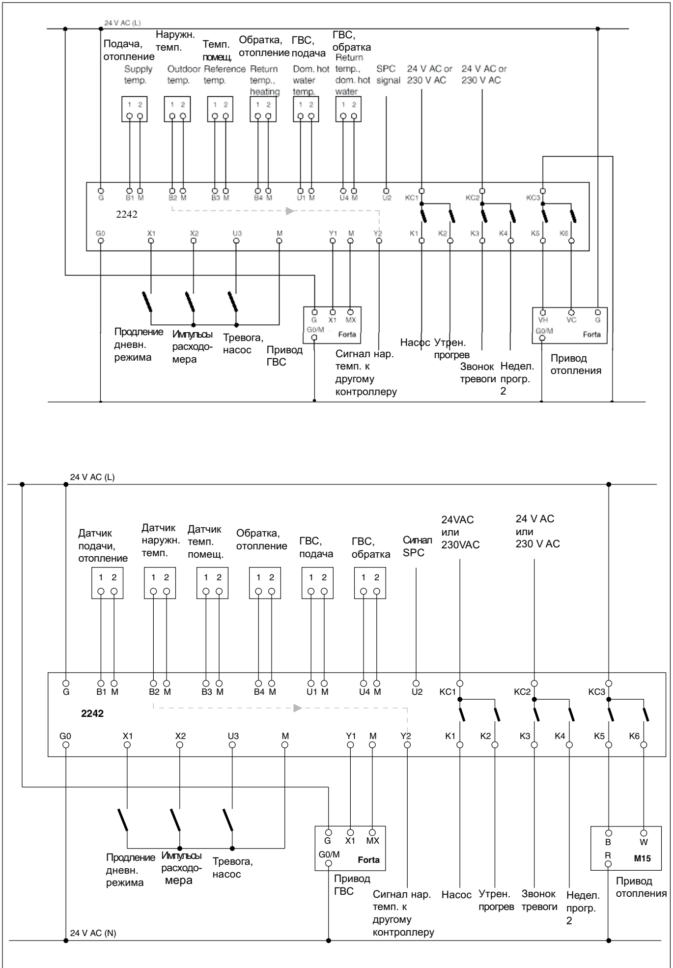
Схемы подключения
