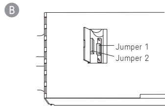
Einstellung für 230 V / 50–60 Hz (Zweiter Jumper unter Gehäuseabdeckung befestigt)
