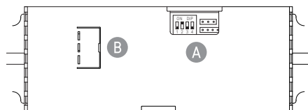
Réglage pour 230 V / 50-60 Hz (Deuxième cavalier fixé sous couvercle boîtier)
