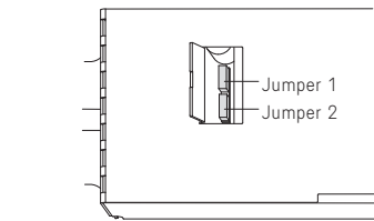
Einstellung für 110 V / 50–60 Hz
