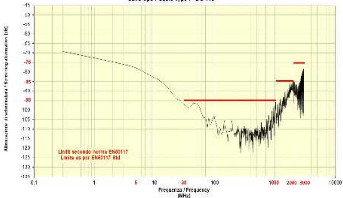
Attenuazione di schermatura / Screening Attenuation Cavo classe A+ / A+ Class Cable Cavo tipo / Cable type : DG 113
