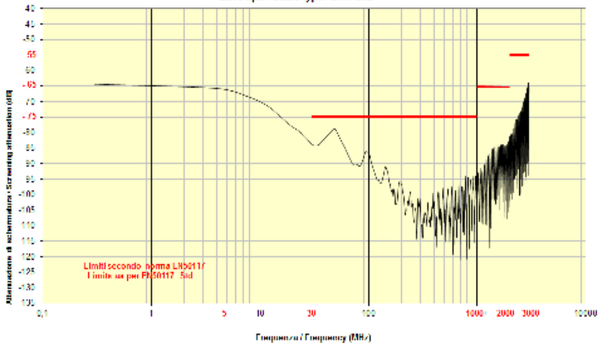
Attenuazione di schermatura / Screening Attenuation Cavo classe B / B Class Cable Cavo tipo / Cable type: SAT703B
