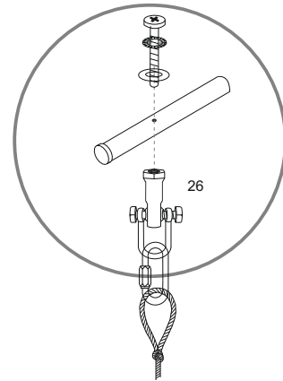
способ крепления качель и лиана
