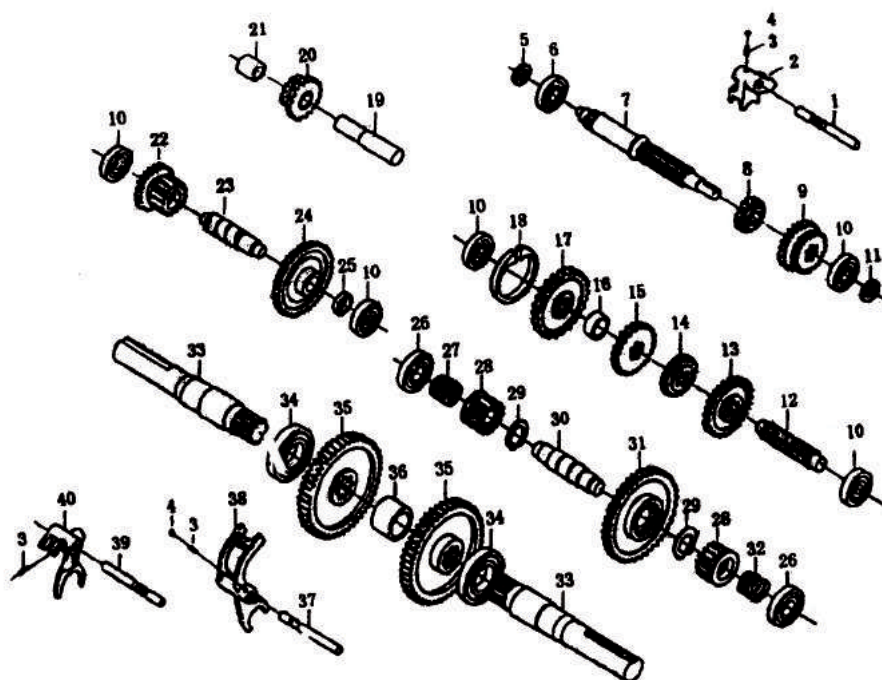
Рис.2. Коробка передач в сборе. (А)
