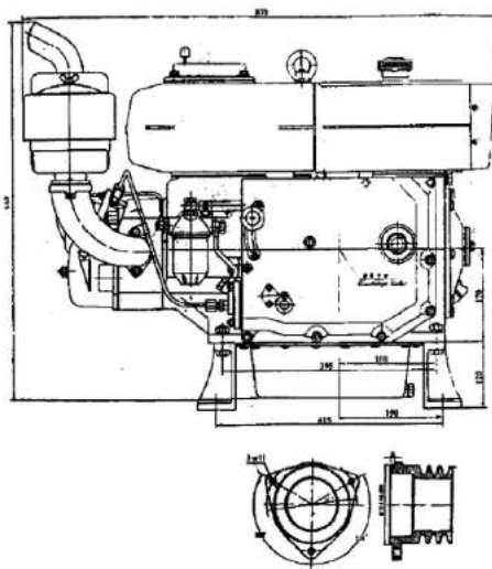
Схематическое изображение двигателя Garden Scout R195
