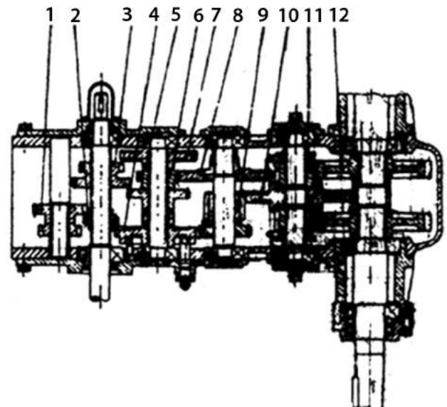
Рис. 4. Коробка передач
