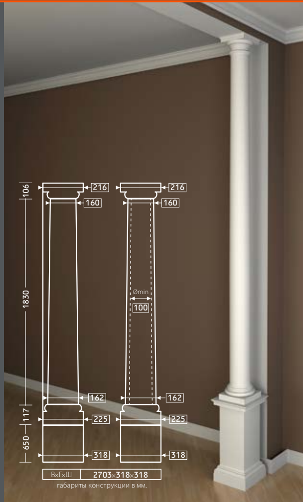
КАПИТЕЛЬ 1.11.008 СТВОЛ 1.12.060
