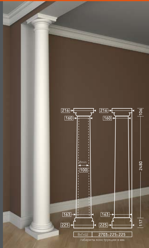
КАПИТЕЛЬ 1.11.008 СТВОЛ 1.12.061
