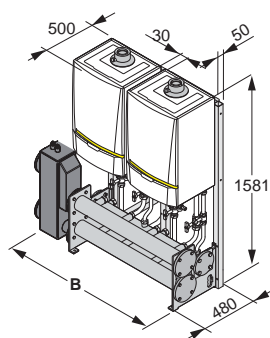
LV: напольный монтаж в один ряд, пример для 2 котлов
