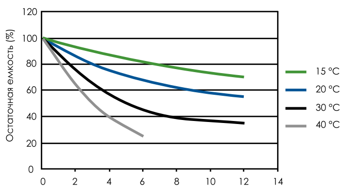
Кривая саморазряда
