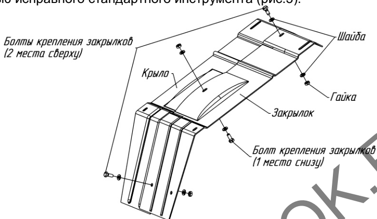
Рис.3. Схема крепления закрывков (дополнительных крыльев)
