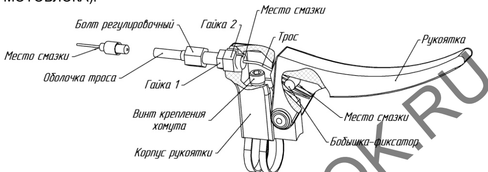
Рис.11. Заделка троса разобращения в рукоятке
