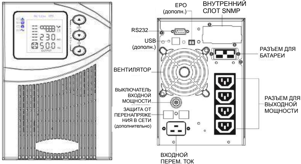
FIG.1 Вид передней панели
