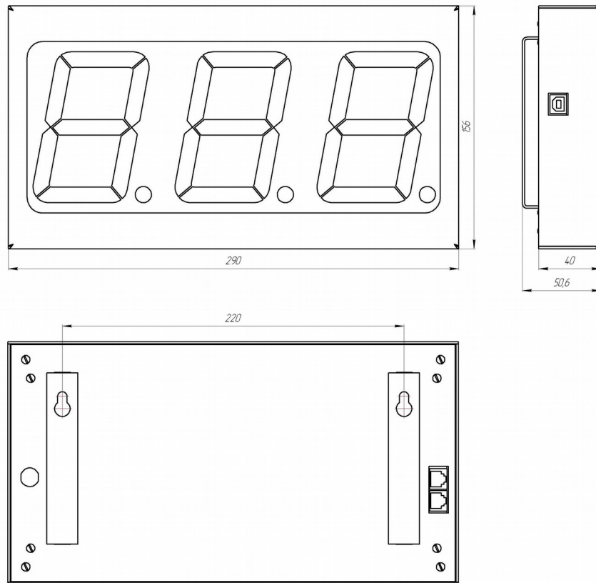
Рис 1. Общий вид, габаритные размеры и элементы конструкции ТИ-D100×3R- DB9-220: 1 - корпус, 2 - крышка корпуса, 3, 4 - разъемы DB-9 интерфейса RS232/RS485, 5 - разъем сетевой \approx 220 В
