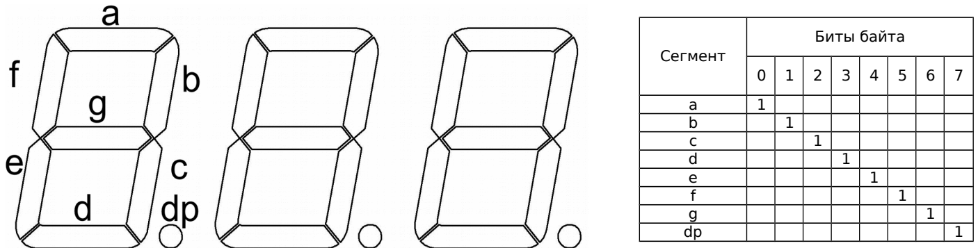
Рис. 6. Табло сегментного типа. Состояние одного сегмента (a, b, c, d, e, f, g, dp) определяет один байт данных (DATA0...DATAN) в соответствии с таблицей включения сегментов (справа)
