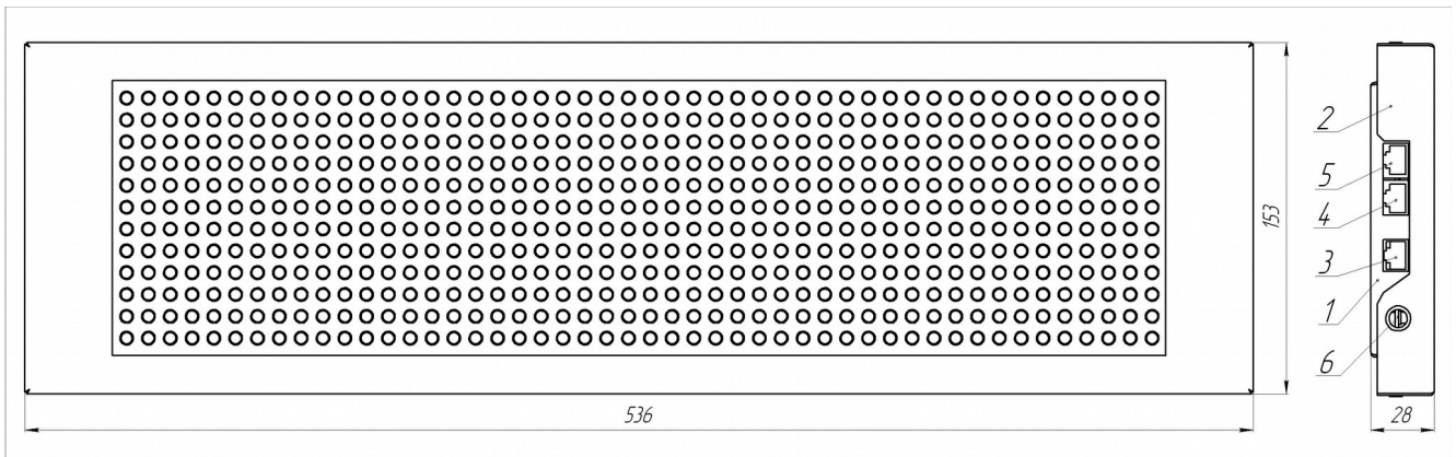
Рис 2. Общий вид, габаритные размеры и элементы конструкции ТИ-M12×48R- RJ45-12: 1 - корпус, 2 - крышка корпуса, 3 - разъем RJ-45 интерфейса Ethernet, 4, 5 - разъемы RJ-45 интерфейса RS232/RS485, 6 - разъем сетевой =12 В.
